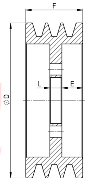
TIPO A - FURO ESPECIAL
