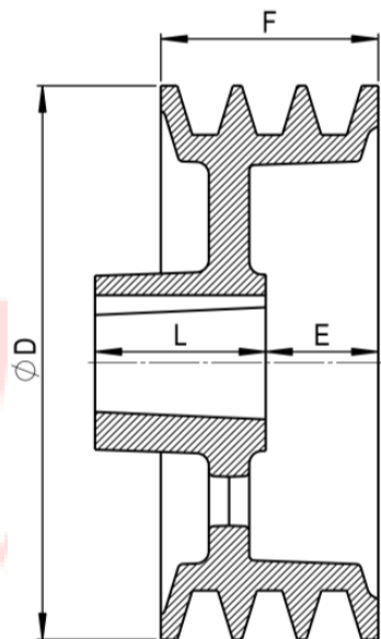
TIPO C2 - ALIVIADA FURO E CHAVETA
